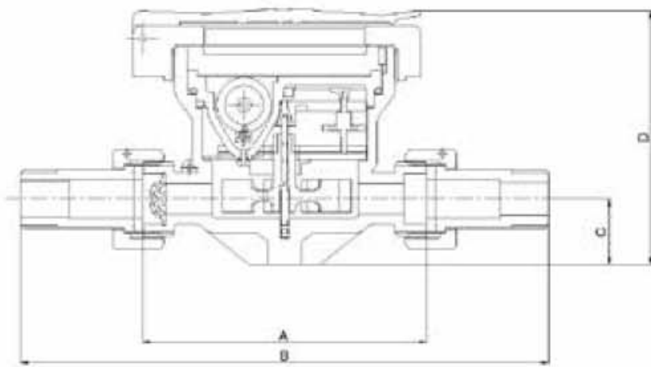
Dimension (mm.)
